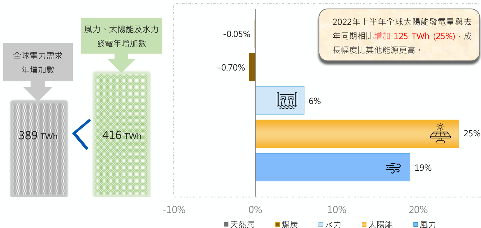
2022年1~6月發電量年變化數
