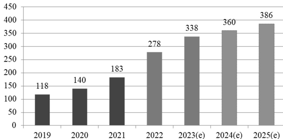
2019-2025 全球太陽能安裝量
