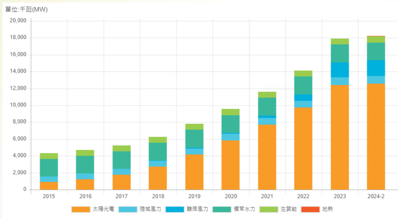
台灣再生能源裝置容量 (2015~2024.2)
